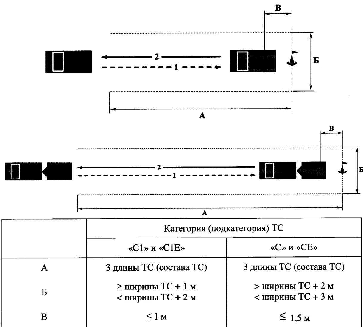
Рисунок 6. Схема и размеры маневра «Прямолинейное движение задним ходом и парковка для погрузки (разгрузки) на погрузочной эстакаде (платформе) (для транспортных средств категорий «С» и «СЕ» и подкатегорий «С1» и «С1Е»)»
