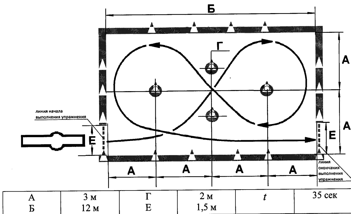
Рисунок 1. Схема и размеры элемента упражнения № 1 – Габаритная восьмерка»
