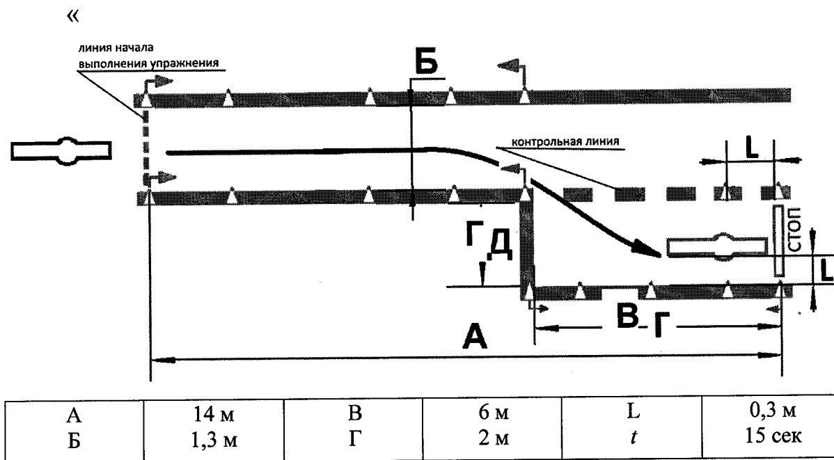
Рисунок 6. Схема и размеры упражнения № 3
