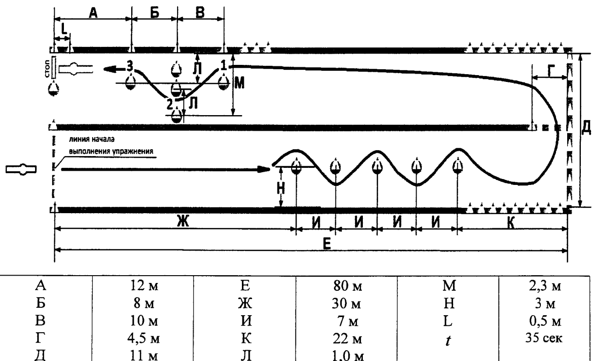
Рисунок 3. Схема и размеры элемента упражнения № 1 – «Скоростное маневрирование»
