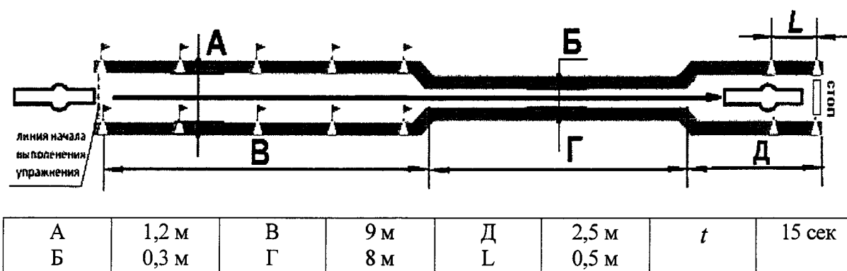
Рисунок 4. Схема и размеры элемента упражнения № 1 - «Габаритный коридор»
